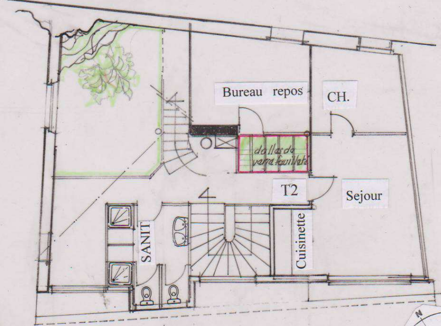
PLAN 1° ETAGE + 3.30
